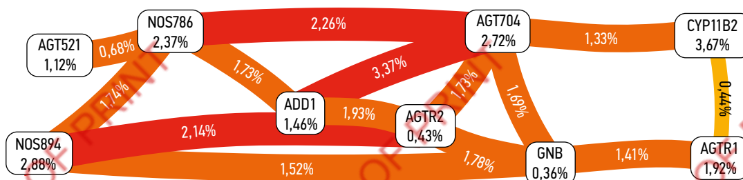
Рис. 3. Граф генетических полиморфизмов (по схеме Фрюхтерман-Рейнгольда). На рёбрах графа представлены значения межгенной энтропии, а на узлах — значения энтропии для каждого отдельного гена. Fig. 3. Graph of genetic polymorphisms (Fruchterman-Reingold scheme). The edges of the graph represent the values of intergenic entropy, and the nodes represent the values of entropy for each individual gene.
